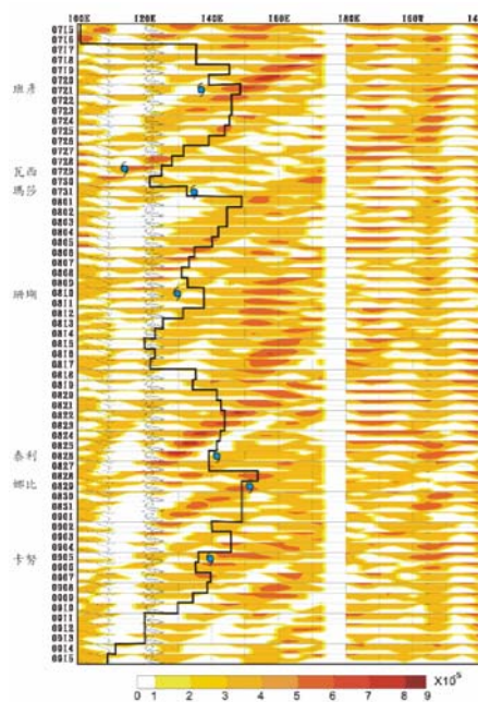
圖三：2005年7月15日至9月15日NCEP絕對渦度的時間序列。黑實線為 10^{\circ}N\sim 20^{\circ}N 平均東西風交界，颱風標記為颱風生成的時間及經度。中太平洋波動進入東西風合流區時，可能有利颱風生成。
