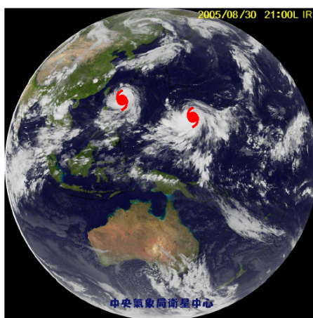
圖一：2005年8月30日衛星雲圖。離台灣較近為泰利颱風，其右後方為娜比颱風。
