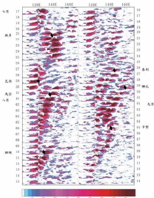
圖二：2005年7月17日至9月14日QickSCAT衛星海表面風 V^2 的時間序列。颱風向西北前進時，向右後方的能量頻散可能有利於下一個擾動生成，並且颱風有連續生成的特性。
