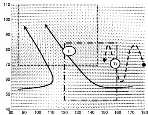
圖五：似季風環流背景場下，渦旋頻散與西行波動交互作用實驗示意圖。標記Ty圓形符號表植入渦旋位置；標記C橢圓形符號表背景場輻合位置；實心圓表波動源位置；虛線箭頭表波動移行方向；實線箭頭表大尺度流場；虛點線方框表擾動渦度區的範圍；點線方框表實驗結果所顯示的範圍。
